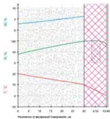
B1 – мокрое утепление по ППС 50/100 мм
